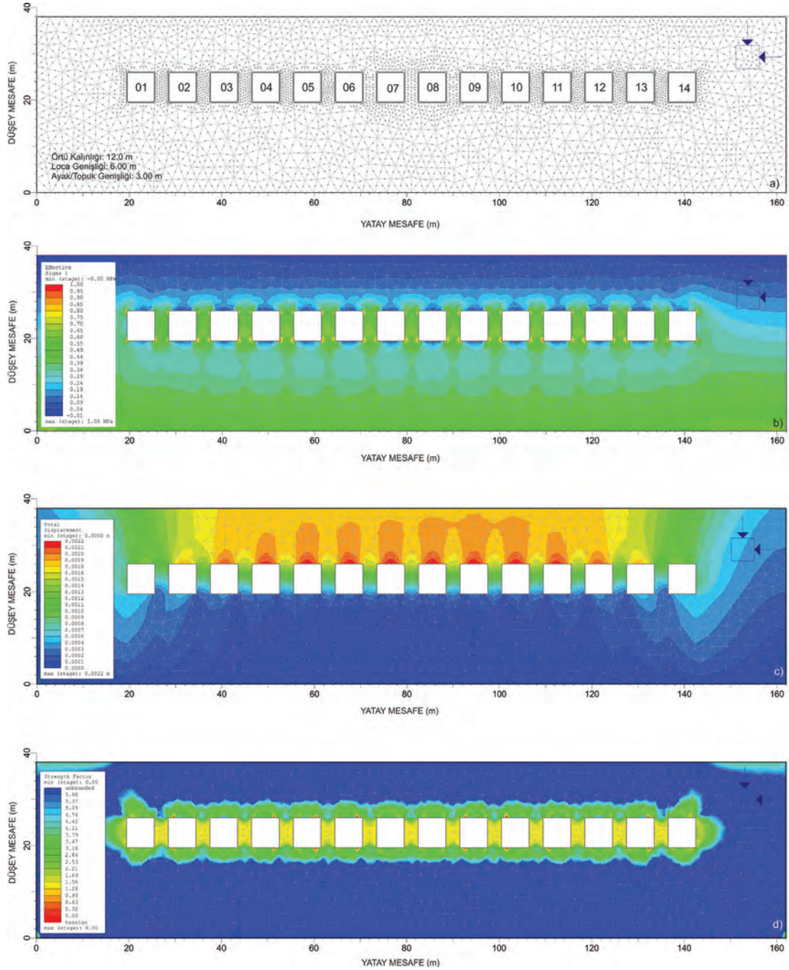
Őekil 6. Kaya oyma depolarda kullanılan genel mimarinin (Model-01) sonlu elemanlar analizi: a) ađ yapısı ve localar, b) efektif dűey gerilme ( s_v ), c) toplam deformasyon, d) dayanım faktörü dađımları.
